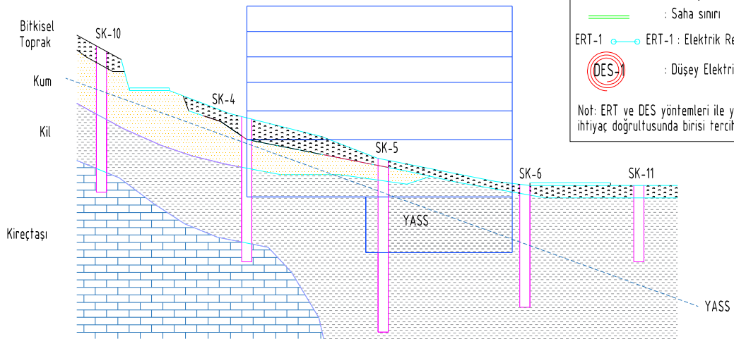
A-A' KESİTİ
