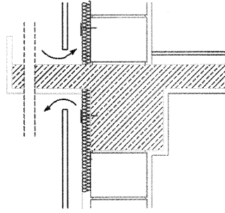
BALKON – DUVAR BIRLESIMI
