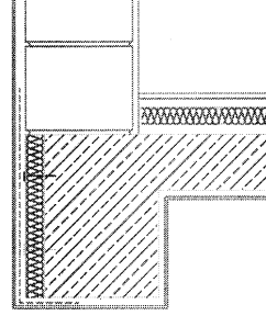
CIKMA – DUVAR BIRLESIMI
