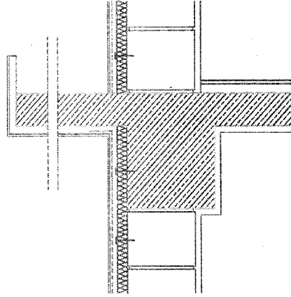
BALKON – DUVAR BIRLESIMI
