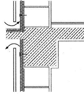
DUSUK DOSEMELI BALKON DETAYI
